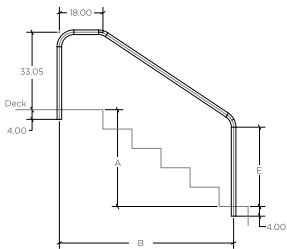
3-Bend Heavy Duty
