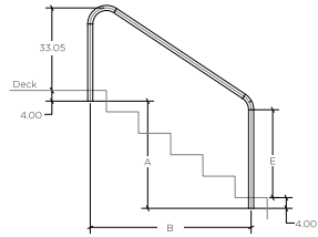
2-Bend Heavy Duty
